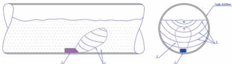
Рис. 4. Установленный датчик скорости в условиях повышенной концентрации взвешенных частиц: 1 – датчик скорости, 2 – покрытие ультразвукового сигнала датчика скорости, 3 – профиль скоростей потока
