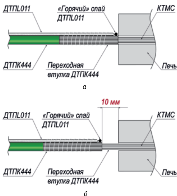
Рис. 6. Этапы эксперимента: а – термопара ДТПК444 полностью («до упора») погружена в печь; б – втулка термопары ДТПК444 отодвинута от стенки печи на 10 мм
