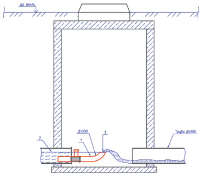
Рис. 8. Наполнение приходящего трубопровода при установке электромагнитного датчика скорости с вертикальным изливом: 1 – датчик скорости, 2 – уровень потока в приходящем трубопроводе, 3 – уровень излива измерительного участка
