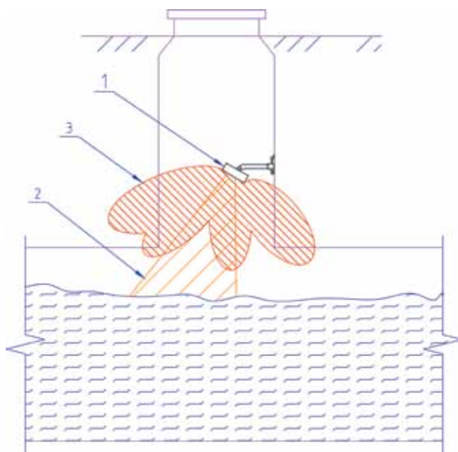
Рис. 2. Условная схема диаграммы направленности основного лепестка и боковых лепестков патч-антенны датчика скорости, установленного в колодце: 1 – датчик скорости, 2 – диаграмма направленности основного лепестка, 3 – диаграмма направленности боковых лепестков
