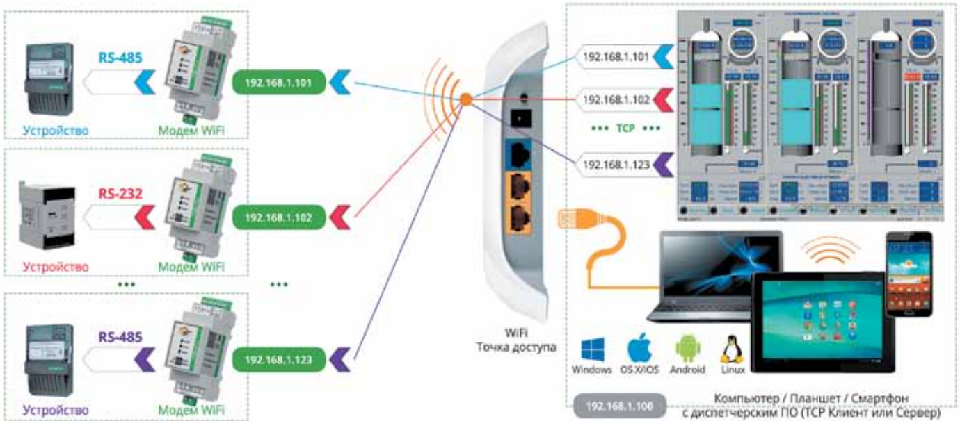
Рис. 4. RS-485/RS-232-устройства, подключенные к модемам PROMODEM Wi-Fi, получают IP-адрес и опрашиваются диспетчерским ПО по TCP-портам
