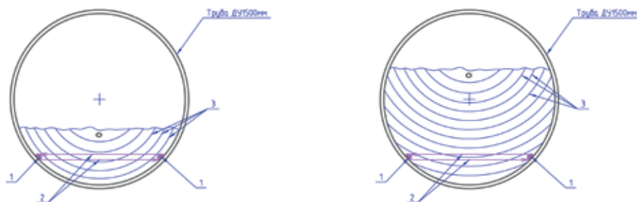
Рис. 6. Неправильная установка ультразвуковых датчиков скорости Transit-Time в зависимости от наполнения трубопровода: 1 – датчик скорости, 2 – ультразвуковой сигнал от датчика к датчику, 3 – профиль скоростей потока
