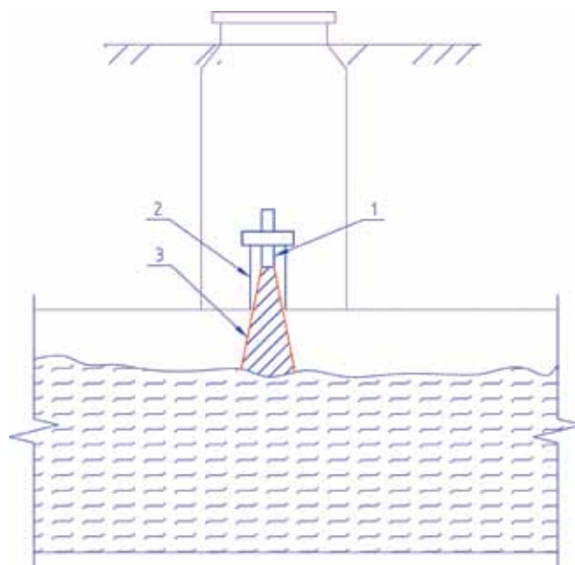
Рис. 9. Расходомер-уровнемер, установленный на безнапорном трубопроводе: 1 – ультразвуковой датчик уровня, 2 – волновод, 3 – ультразвуковое излучение
