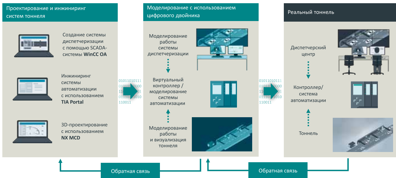
Рис. 7. Цифровая цепочка создания систем автоматизации и диспетчеризации тоннеля
