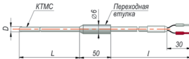
Рис. 3. Конструктивное исполнение ОВЕН ДТПХхх4
