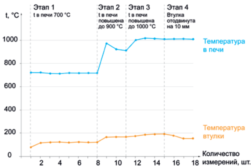
Рис. 7. График изменения температур в печи и на переходной втулке
