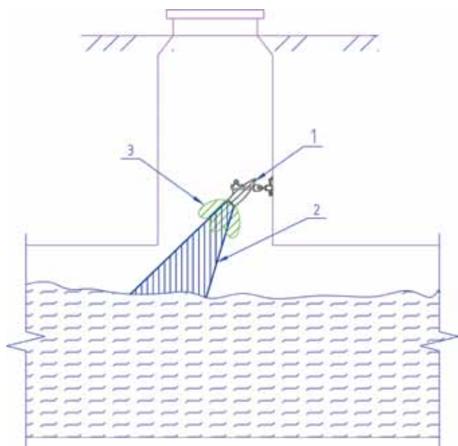
Рис. 1. Условная схема диаграммы направленности основного лепестка и боковых лепестков рупорной антенны датчика скорости, установленного в канализационном колодце: 1 – датчик скорости, 2 – диаграмма направленности основного лепестка, 3 – диаграмма направленности боковых лепестков
