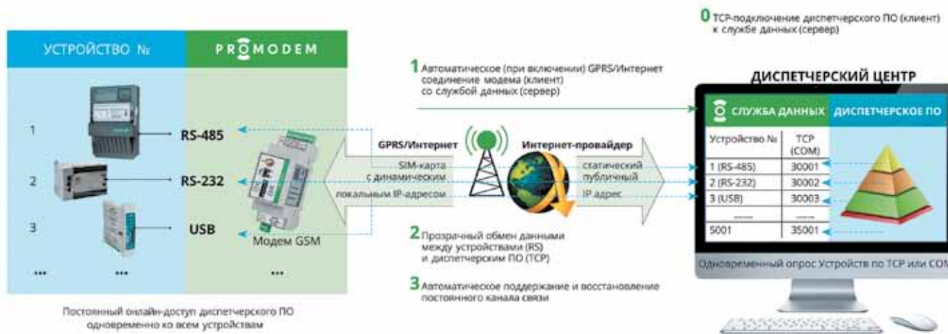
Рис. 2. Одновременный онлайн-доступ диспетчерского ПО ко всем устройствам, подключенным к модемам (режим «клиент»)
