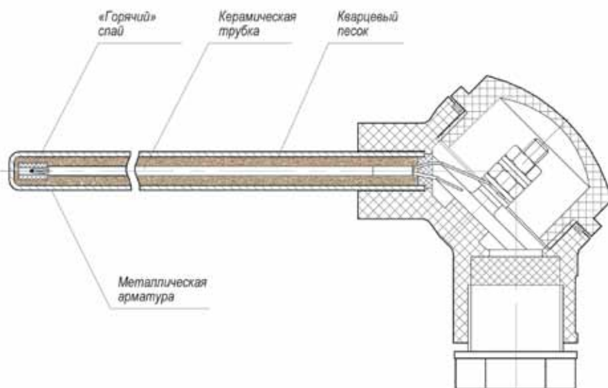
Рис. 1. Термоэлектрический преобразователь
