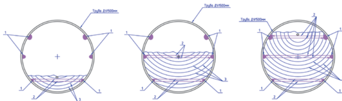
Рис. 7. Правильная установка ультразвуковых датчиков скорости Transit-Time в зависимости от наполнения трубопровода: 1 – датчик скорости, 2 – ультразвуковой сигнал от датчика к датчику, 3 – профиль скоростей потока
