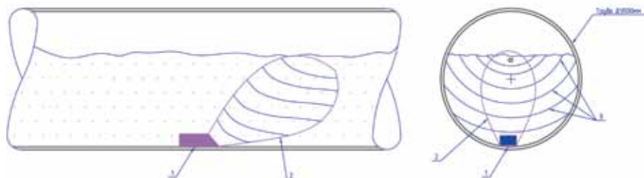
Рис. 3. Установленный датчик скорости в условиях умеренной концентрации взвешенных частиц: 1 – датчик скорости, 2 – покрытие ультразвукового сигнала датчика скорости, 3 – профиль скоростей потока
