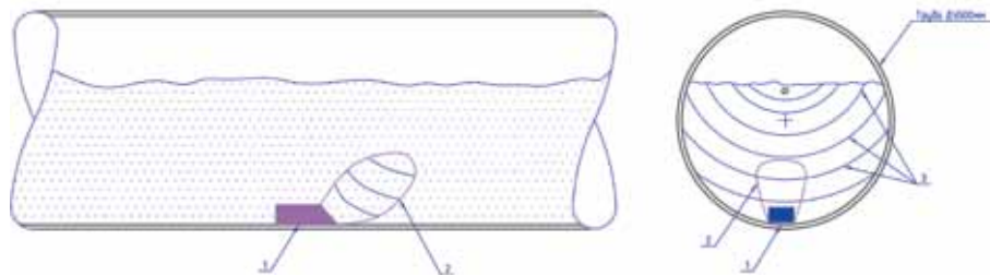
Рис. 5. Установленный датчик скорости в условиях высокой концентрации взвешенных частиц: 1 – датчик скорости, 2 – покрытие ультразвукового сигнала датчика скорости, 3 – профиль скоростей потока
