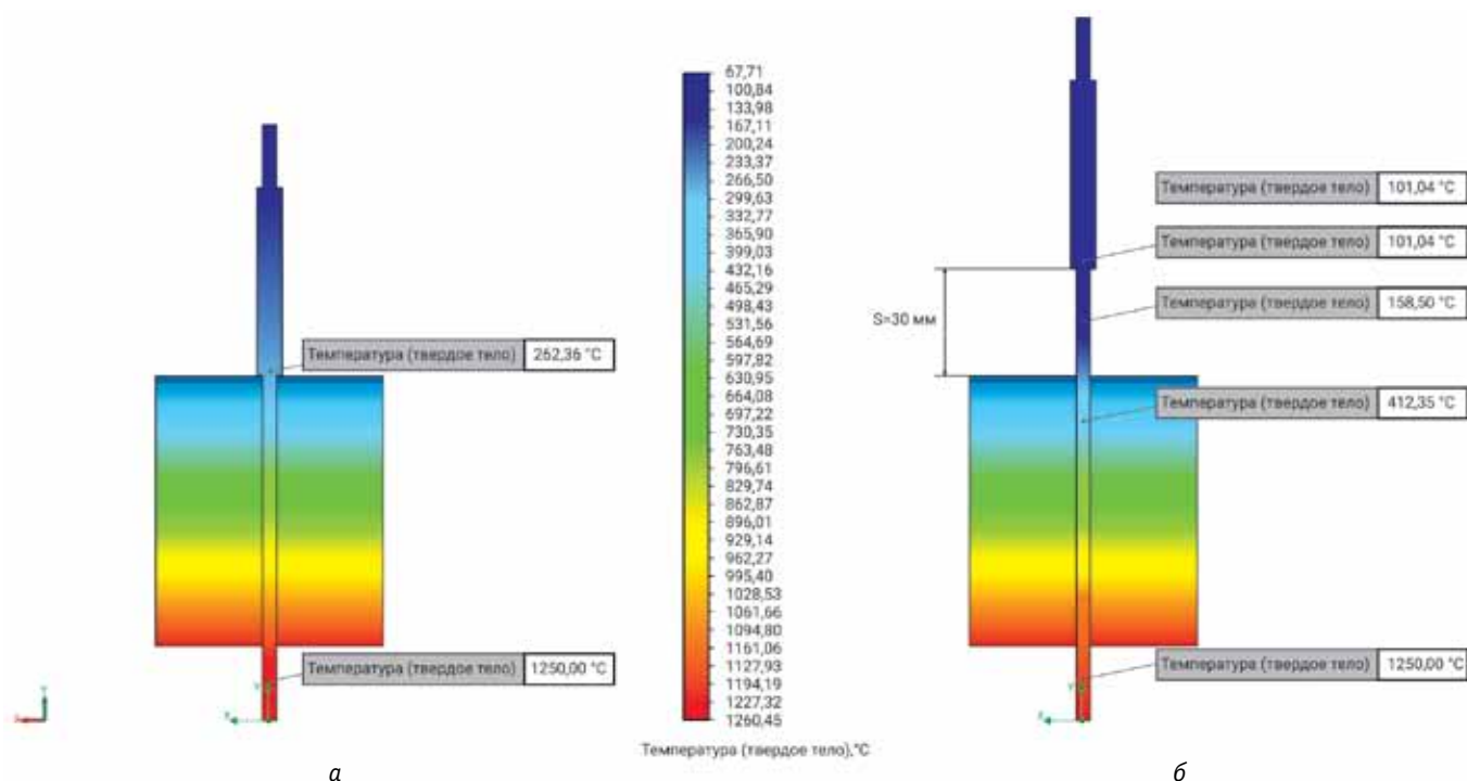
Рис. 4. Варианты моделирования условий эксплуатации датчика: а – модель № 1. Распределение температур по длине датчика, датчик полностью погружен в печь;
