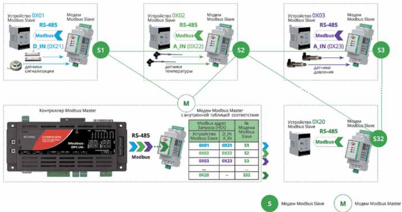
Рис. 3. Беспроводной опрос Modbus-master-контроллером Modbus-slave-устройств и датчиков по радиоканалу ZigBee – замена проводной шины RS-485
