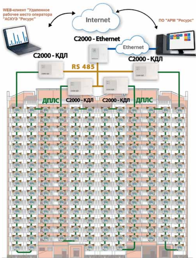
Рис. 2. Схема построения АСКУЭ «Ресурс»: учет водоснабжения, г. Серпухов
