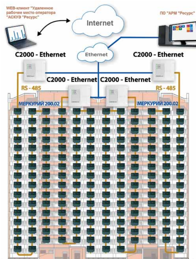
Рис. 3. Схема построения АСКУЭ «Ресурс»: учет электроэнергии, г. Серпухов
