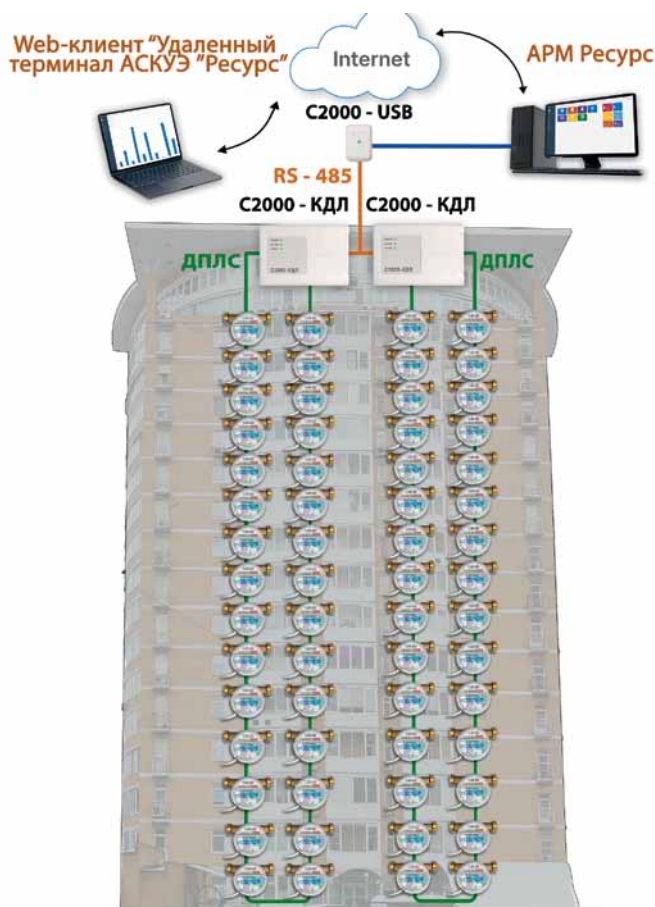
Рис. 5. Схема построения АСКУЭ «Ресурс»: учет водоснабжения, г. Москва
