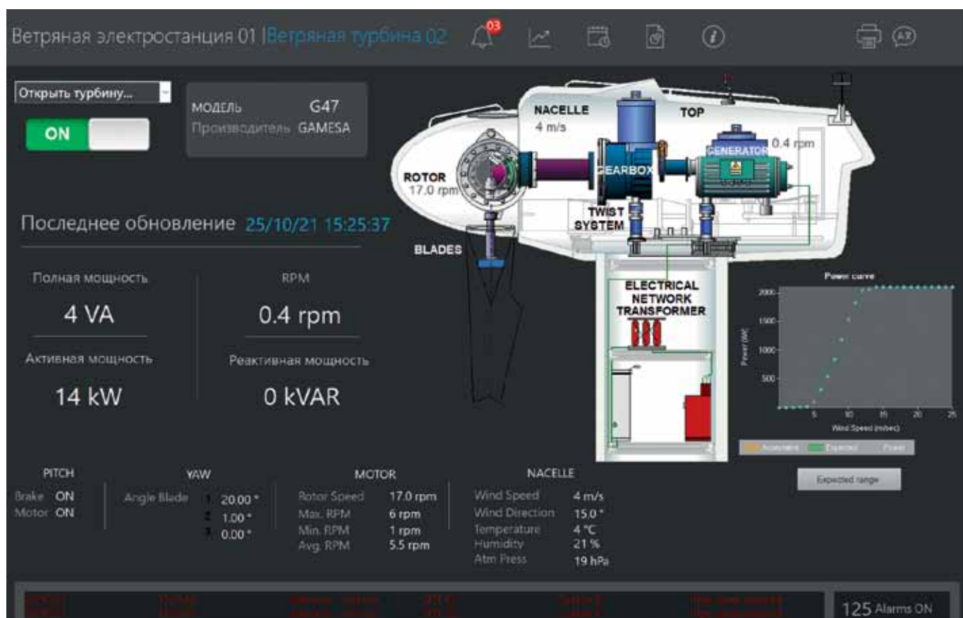
Рис. 1. Пример мнемосхемы SCADA PcVue
