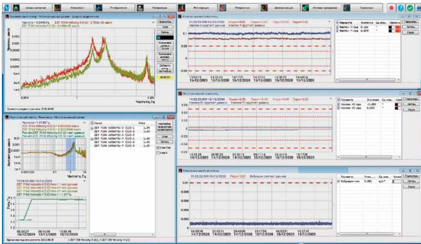
Рис. 6. Динамические характеристики бизнес-центра в программе «Просмотр трендов» компании ZETLAB
