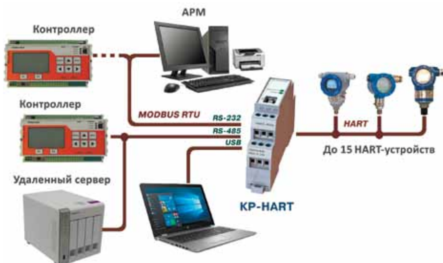
Рис. 1. Система сбора данных, построенная на базе контроллера КР-HART
